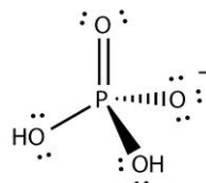
Pi
