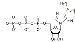
ATP
